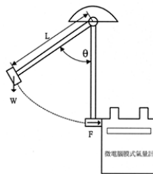
圖 1 衝擊測試
