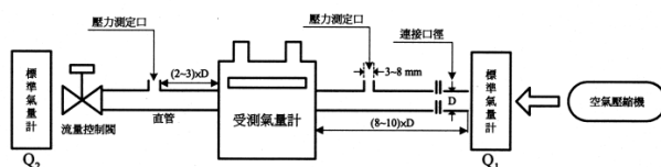
圖 B.2 氣量計測試配置參考圖例
