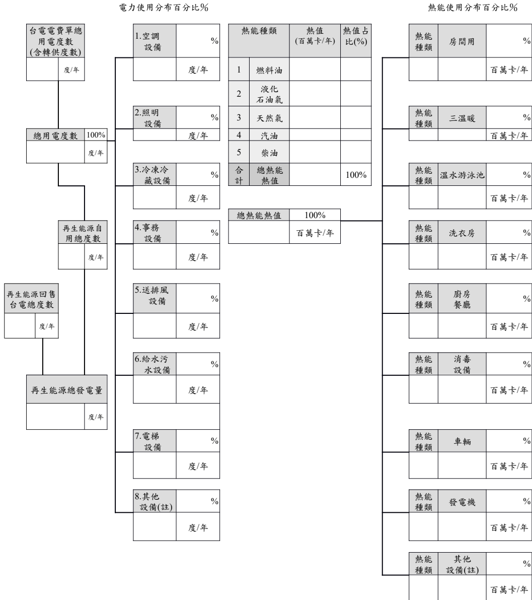
電能用量平衡圖
