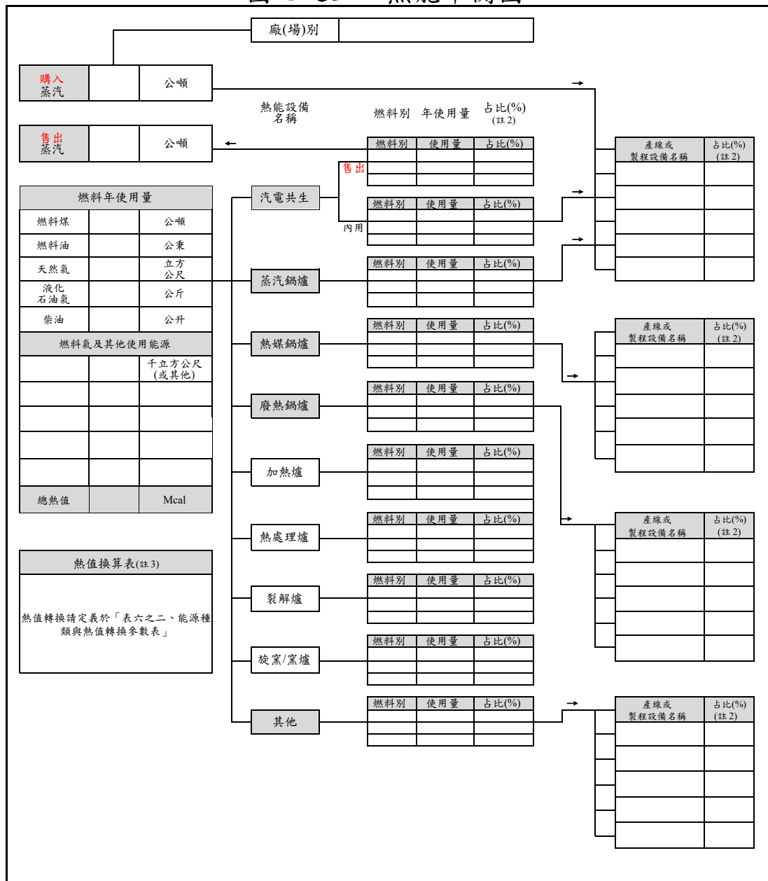
圖七之三、熱能平衡圖
