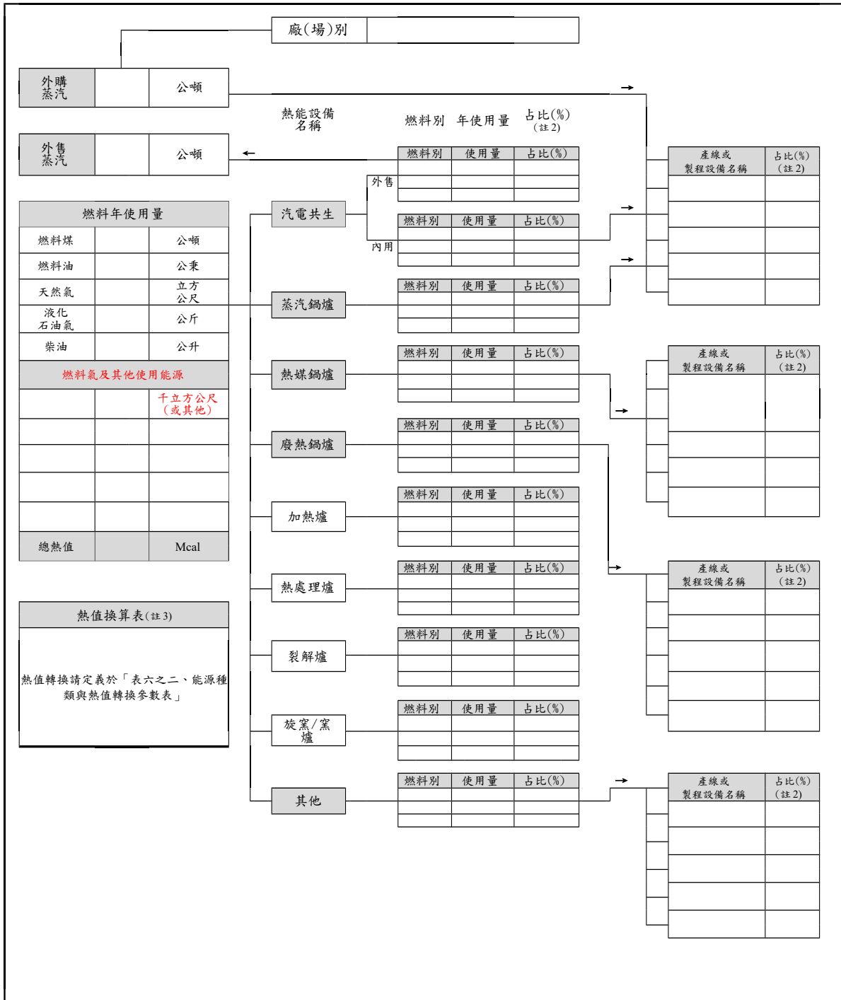
圖七之三、熱能平衡圖
